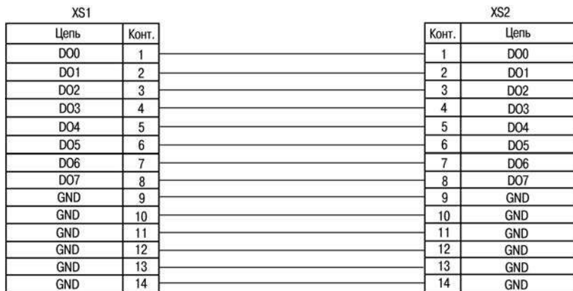
Рисунок В.3 – Схема кабеля для подключения дискретных выходов КС19
